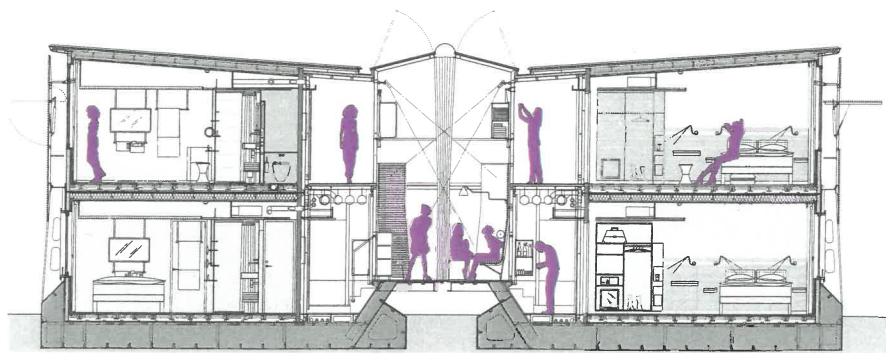
Coupe chambres.
